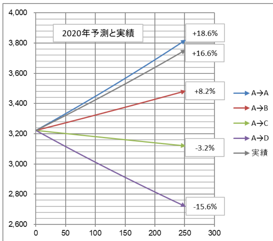
2020 年の終値の四つのパターン予測と実績
